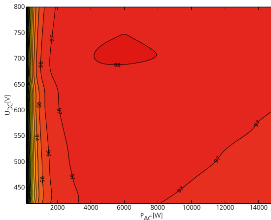
Wirkungsgradkennlinie Powador 18.0 TL3
